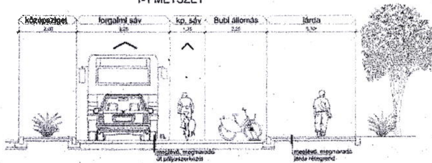
1-1 METSZET
