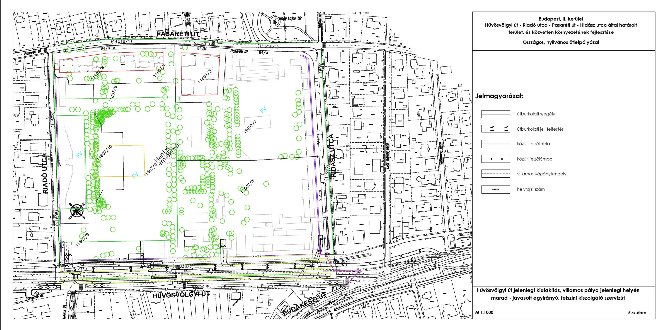
5. ábra Húvösvölgyi út jelenlegi kialakítás, villamos pálya jelenlegi helyén marad – javasolt egyirányú, felszíni kiszolgáló szervízút
